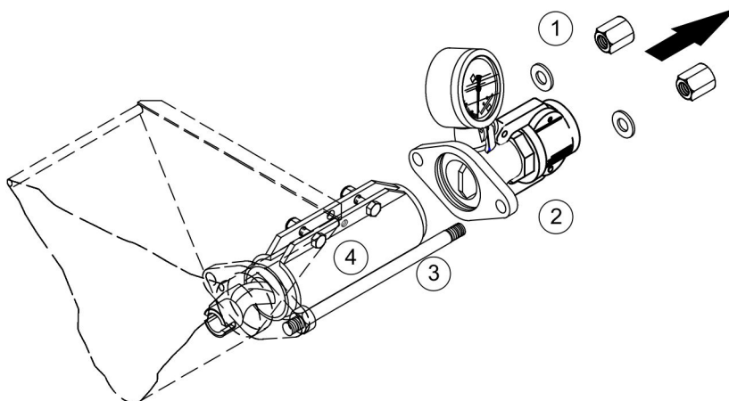
Figura 43: Desmontar a bomba de parafuso semfim
