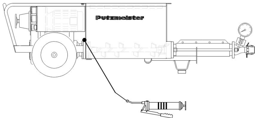
Figura 39: Lubrificar a máquina
