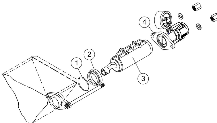
Figura 45: Montar a bomba de parafuso semfim
