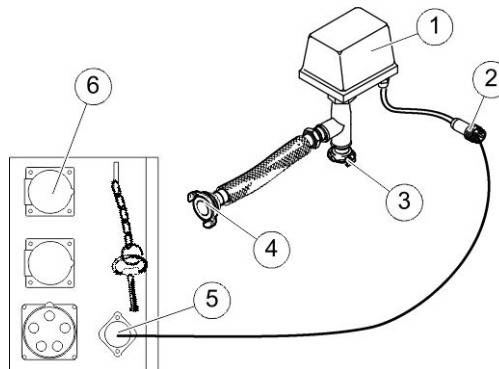
Figura 30: Ligar o controlo remoto do ar comprimido
