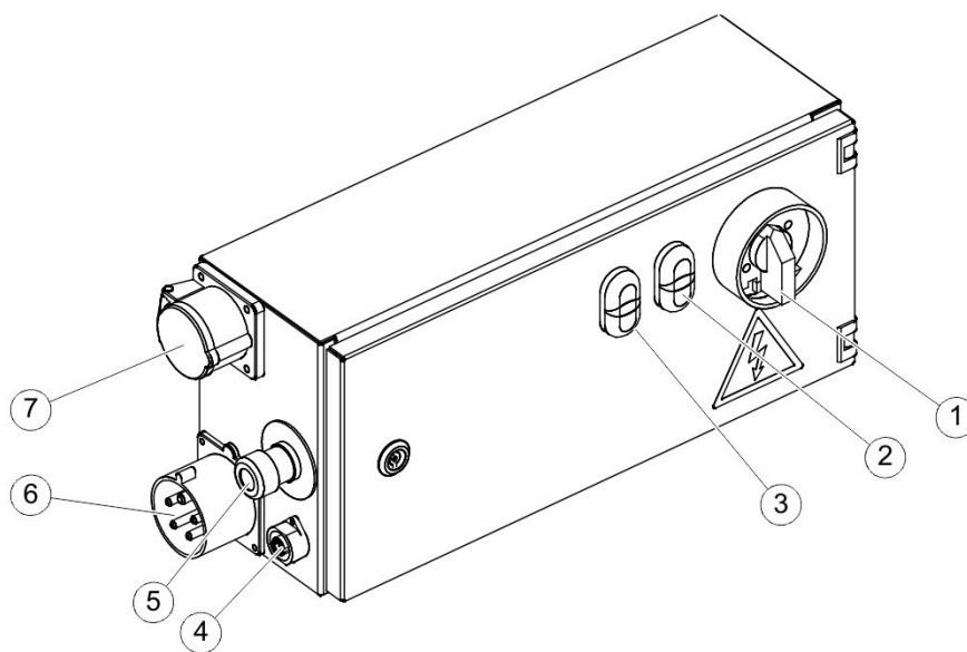
Figura 8: Armário de comando
