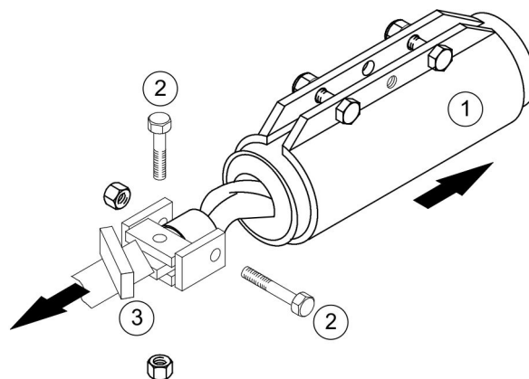
Figura 44: Retirar a bomba de parafuso semfim (são possíveis diferentes versões)
