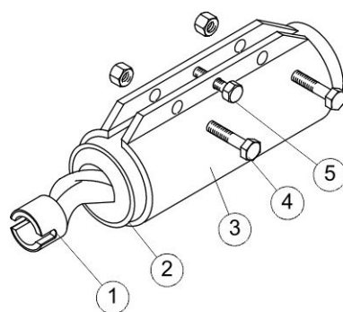
Figura 42: Substituição do semfim de bombagem
