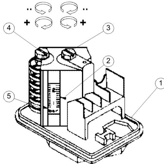
Figura 41: Ajustar o pressóstato
