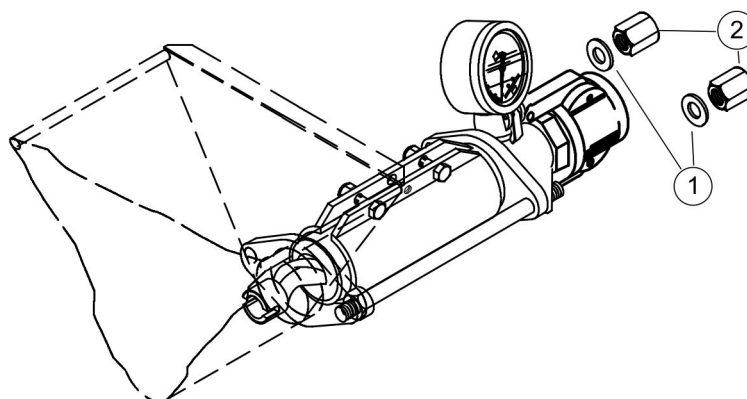
Figura 47: Apertar as porcas de aperto
