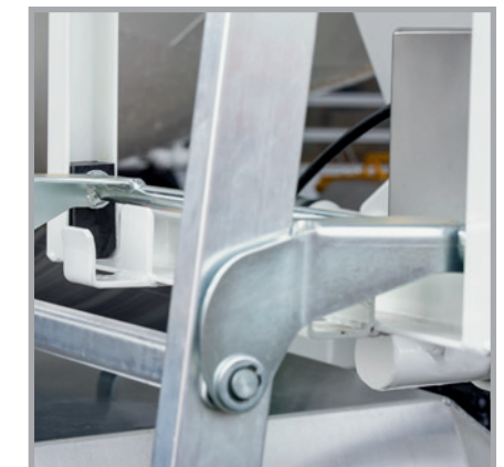
Sicheres und komfortables Handling der Leiter durch eine durchdachte Konstruktion der seitlichen Halterkonturen.
