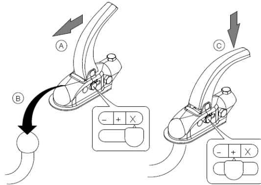
Abbildung 21: Ankuppeln der Kugelukplung
