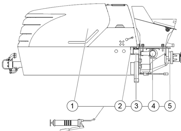
Abbildung 45: Übersicht Schmierstellen
