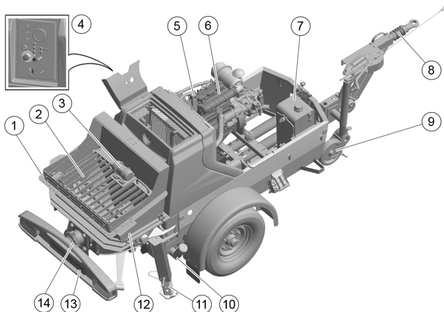
Abbildung 4: Abbildung zeigt Diesel Ausführung (ohne Haube)
