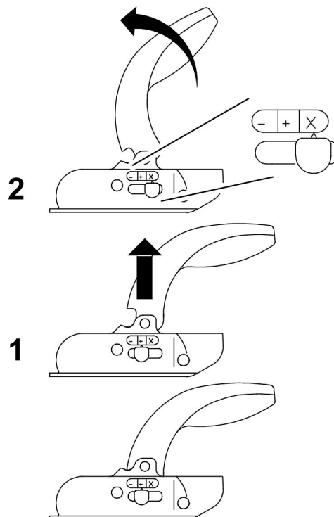
Abbildung 24: Kugelpkupplung abkuppeln
