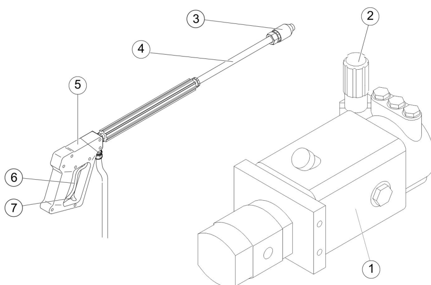
Abbildung 13: Übersicht Hochdruckreiniger
