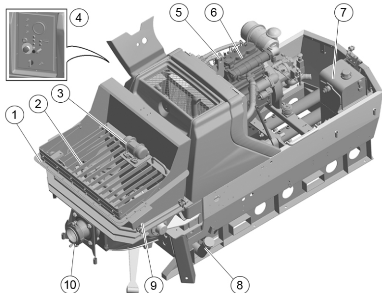
Abbildung 5: Abbildung zeigt Diesel Ausführung (ohne Haube)
