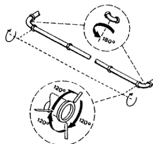
Abbildung 55: Förderrohre und -bögen regelmäßig drehen
