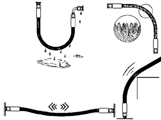
Abbildung 50: Schäden an Hydraulikschlauchleitungen
