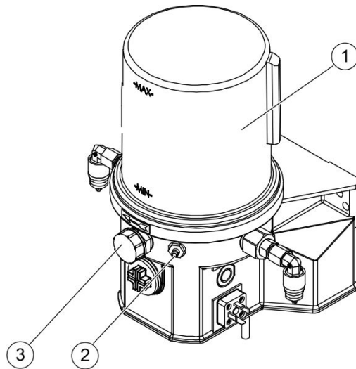
Abbildung 46: Fettzentralschmierung
