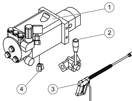
Abbildung 57: Hochdruckreiniger
