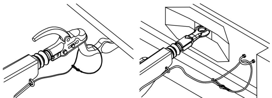
Abbildung 26: Anhängervorrichtung mit Kugelpkupplung oder Zugöse
