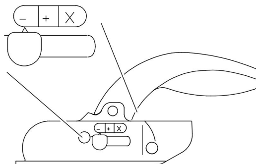
Abbildung 23: Kugelkupplung Stellung „fehlerhaft geschlossen“
