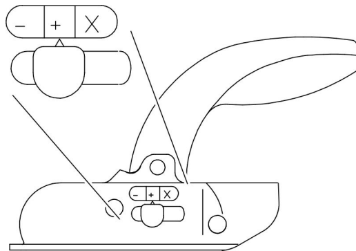
Abbildung 22: Kugelkupplung Stellung „korrekt geschlossen“
