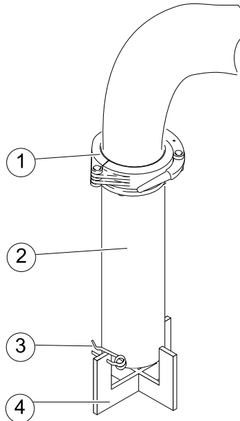
Abbildung 37: Montierter Fangkorb
