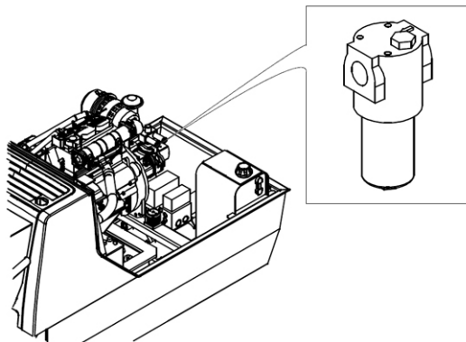
Abbildung 49: Rücklaufgrobfilter im Motorinnenraum
