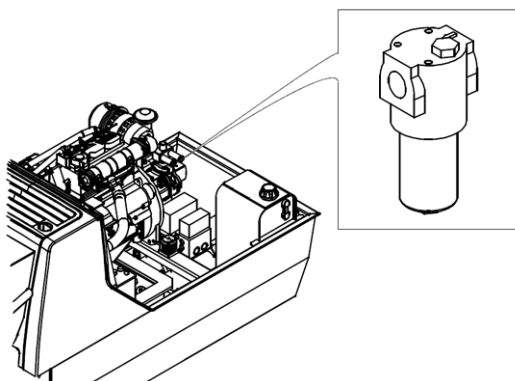
Figure 49: Filtre grossier de retour dans le compartiment moteur interne
