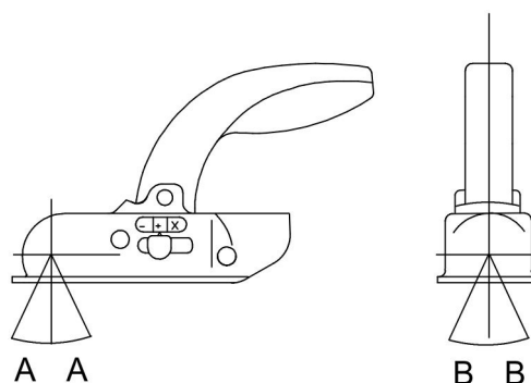
Figure 25: Plage de pivotement du dispositif d'attelage à boule
