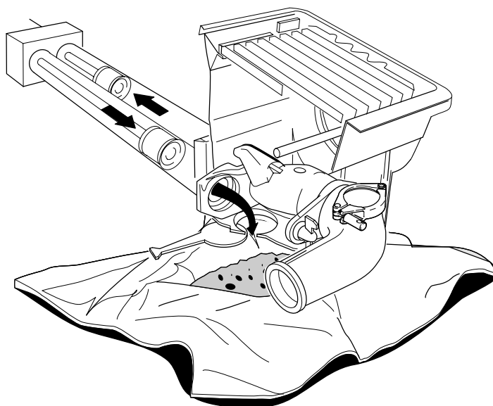
Figure 33: Placer la bâche endessous
