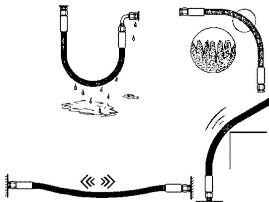
Figure 50: Dommages au niveau des flexibles hydrauliques
