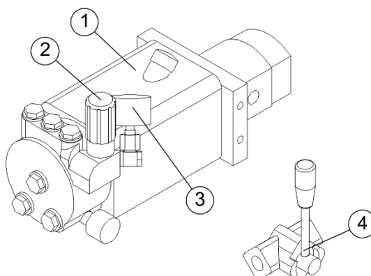
Figure 42: Nettoyeur haute pression - Réglage du levier
