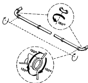
Figure 55: Rotation régulière des tuyaux et coudes de refoulement
