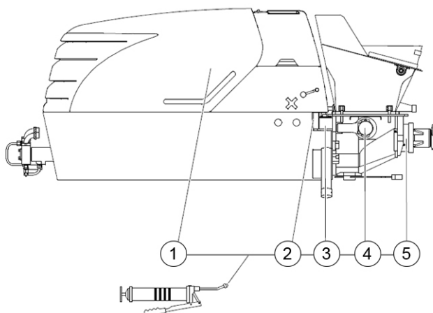
Figure 45: Aperçu des points de lubrification
