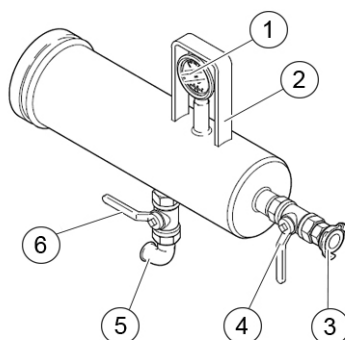
Figure 38: Montage de l'embout de nettoyage
