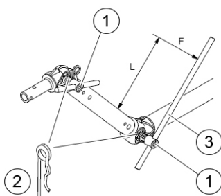
Figure 19: Dispositif d'attelage (différentes versions possibles)
