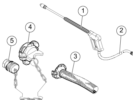
Figure 41: Nettoyeur haute pression - plusieurs versions possibles
