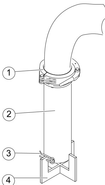
Figure 37: Panier récepteur monté
