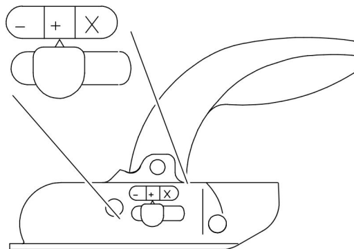
Figure 22: Dispositif d'attelage à boule en position «correctement fermé»
