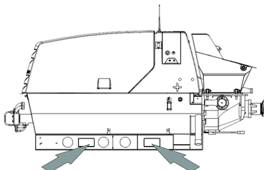
Figure 14: Possibilité d'introduction des fourches d'un chariot élévateur
