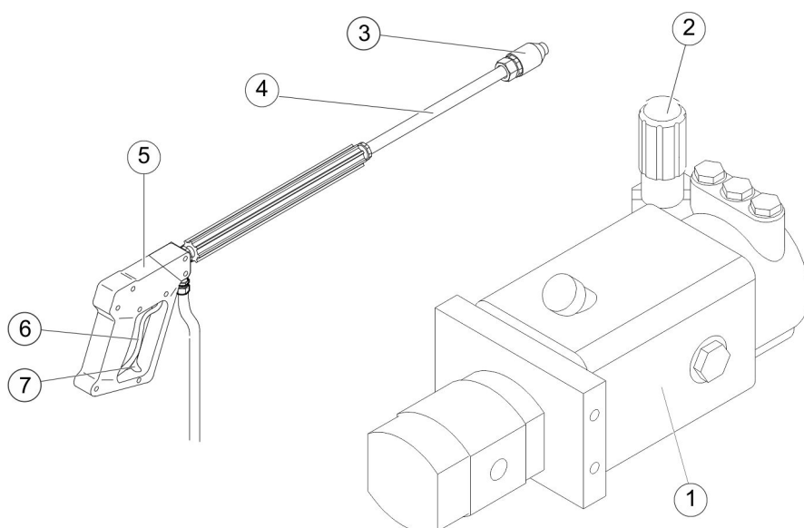
Figure 13: Vue d'ensemble du nettoyeur haute pression
