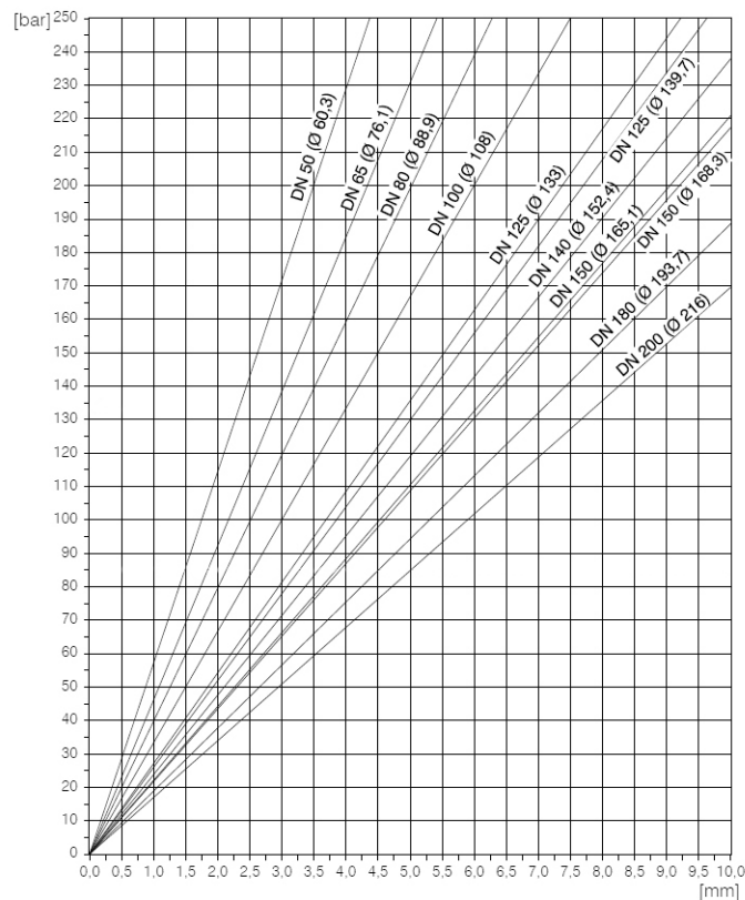
Figure 56: Tableau épaisseurs de paroi
