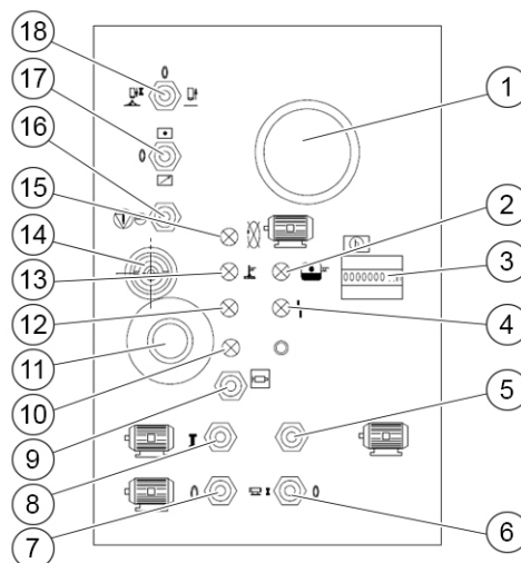
Figure 9: Machine avec moteur d'entraînement électrique
