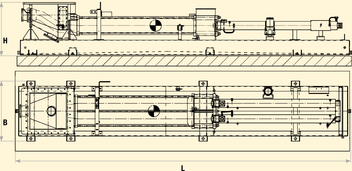
KOS Dickstoffpumpe, Abb. beispielhaft
