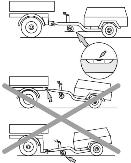
Şekil 35: Makineyi yatay pozisyonda takın
