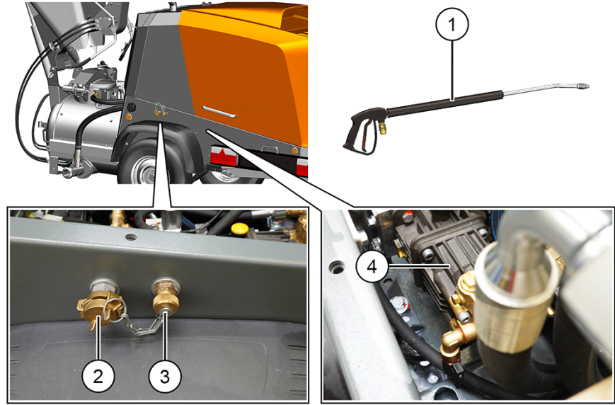
Şekil 20: Yüksek basınçlı temizleyici
