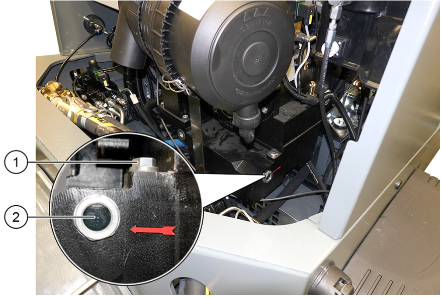
Şekil 74: Kompresör yağı için gözetleme camı
