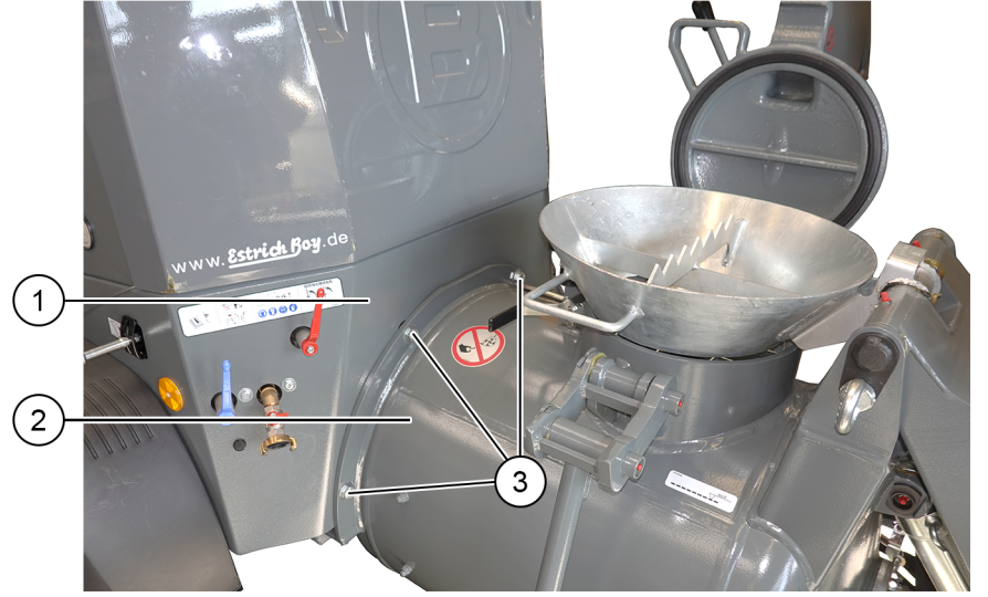
Şekil 94: Karıştırma haznesi vidalı bağlantısı, çerçeve
