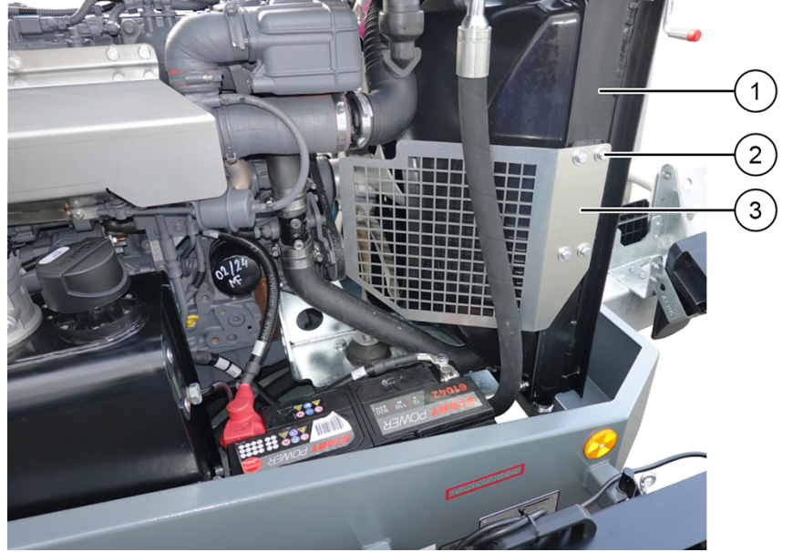
Şekil 90: Radyatörün sağındaki koruma kafesi
