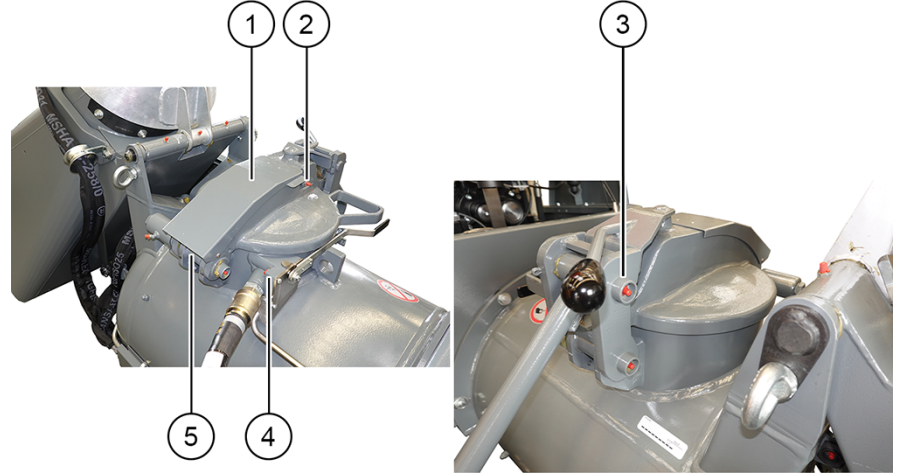
Şekil 79: Karıştırma haznesi kapağının yağlama noktaları
