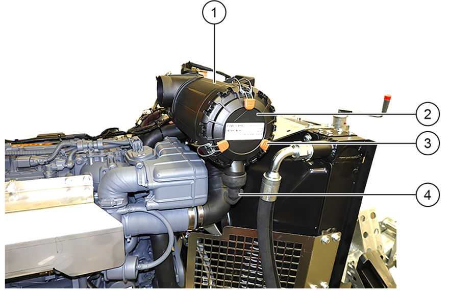
Şekil 81: Hava filtresi muhafazası
