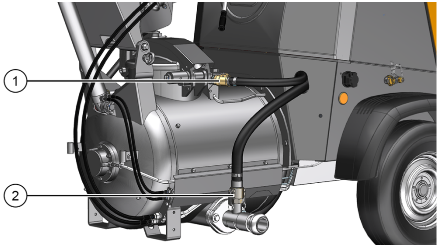
Şekil 87: Üst hava, besleme havası hattı
