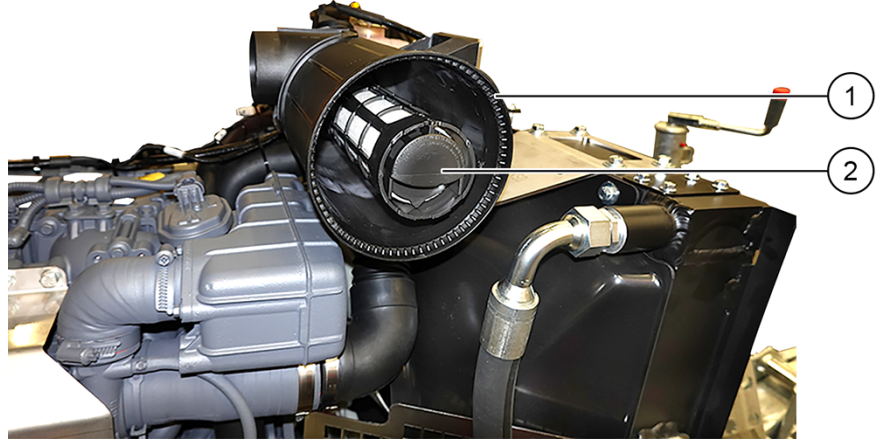
Şekil 83: Tahrik motoru hava filtresinin filtre elemanı
