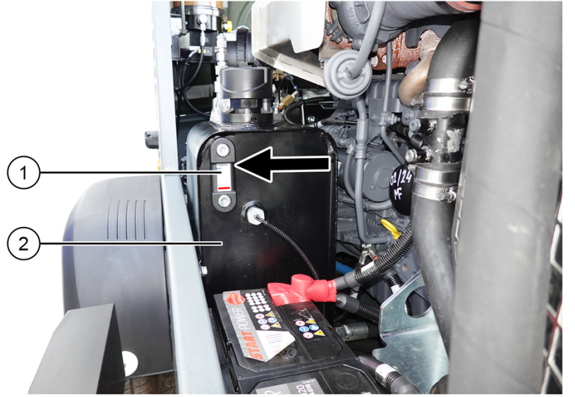
Şekil 73: Hidrolik yağı deposu
