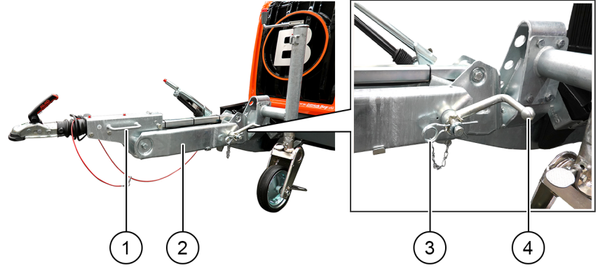
Şekil 37: Yükseklik ayarı AHK
