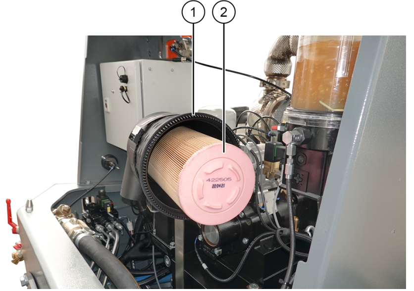
Şekil 85: Kompresör hava filtresi
