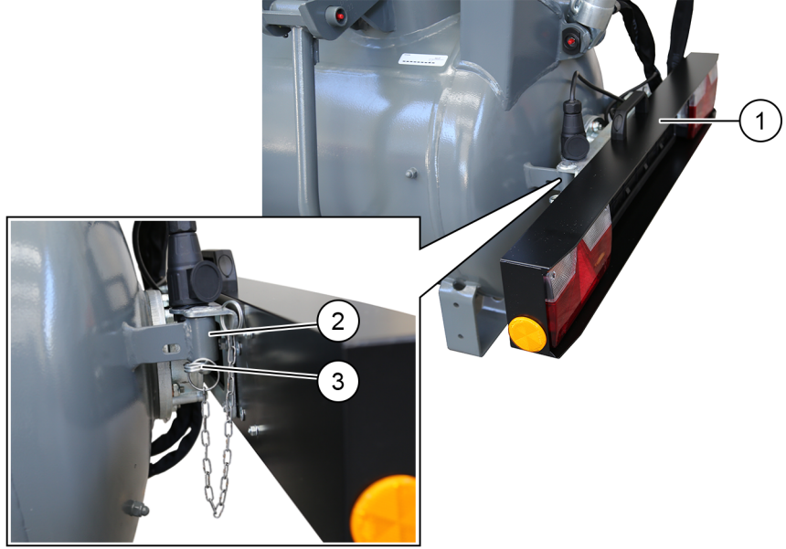
Şekil 33: Aydınlatma tertibatı
