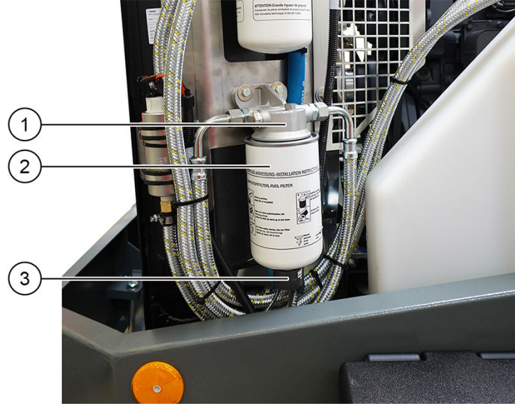
Şekil 91: Yakıt ön filtresi
