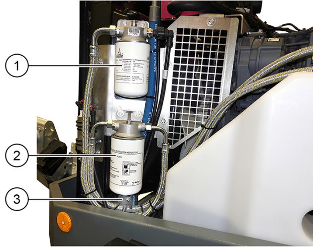
Şekil 92: Yakıt filtresi
