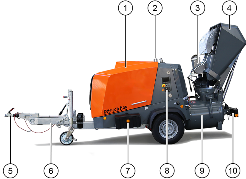
Şekil 3: EstrichBoy
