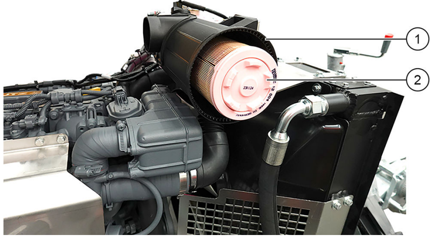
Şekil 82: Tahrik motoru hava filtresinin filtre elemanı
