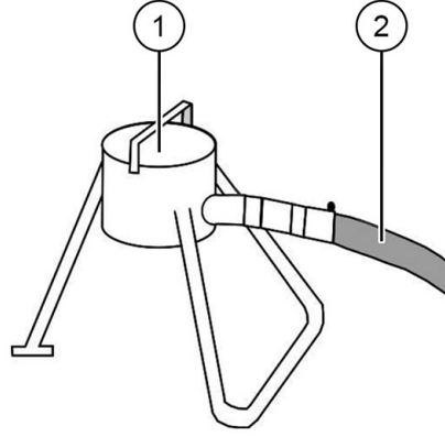
Şekil 67: Üç ayağı bağlama
