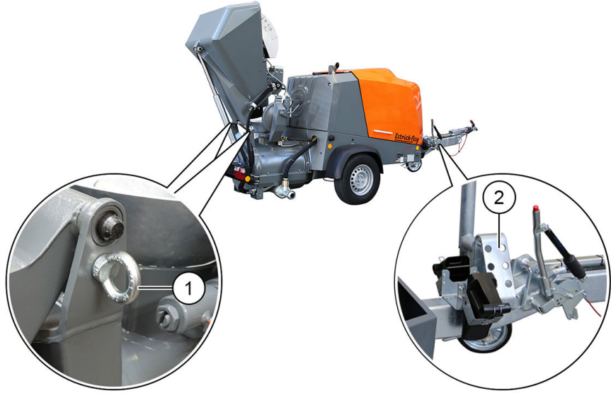
Şekil 30: Besleyicili (B, BS) makine için nakliye emniyeti
