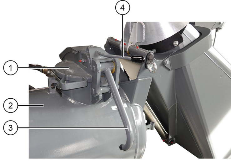
Şekil 65: Karıştırma haznesi kapağı
