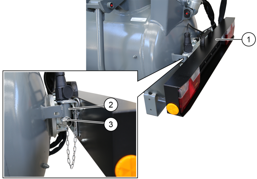
Şekil 42: Aydınlatma tertibatı
