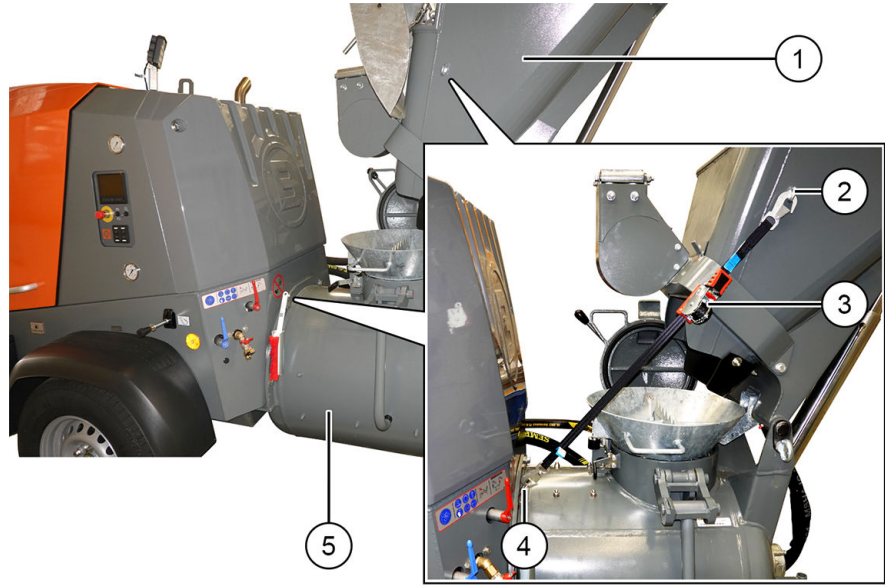
Şekil 28: Besleyici nakliye emniyeti
