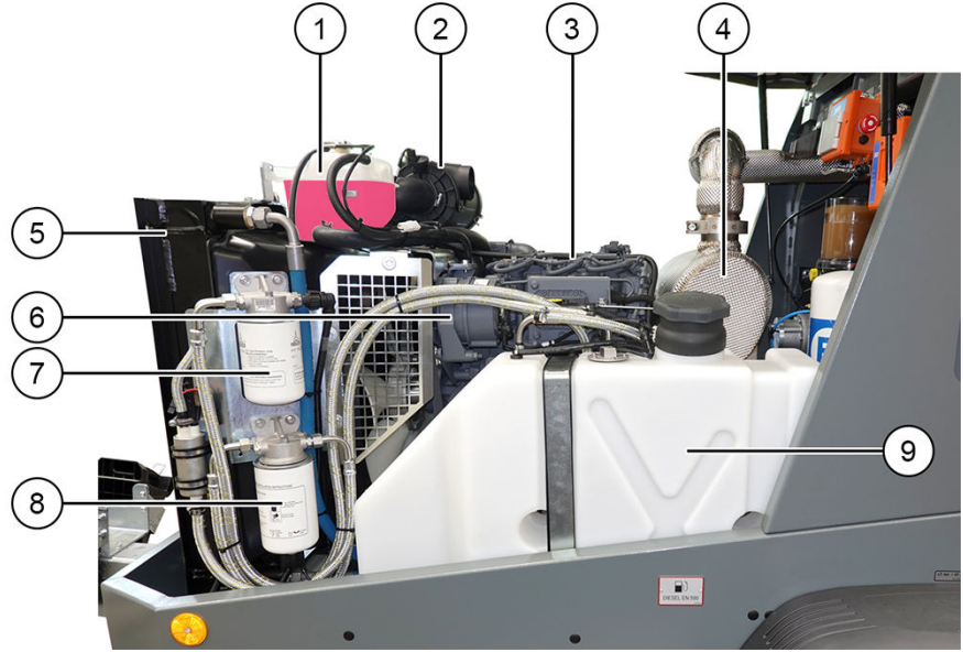
Şekil 8: Soldan görünüm
