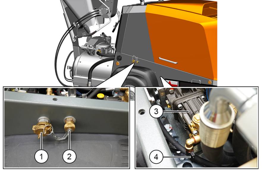
Şekil 93: Yüksek basınçlı su pompası (opsiyon)
