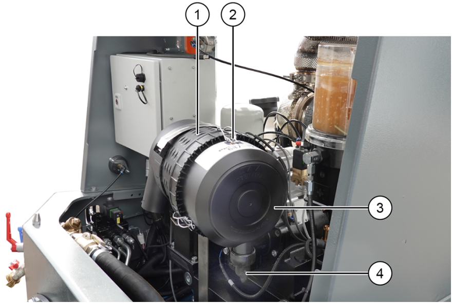
Şekil 84: Kompresör hava filtresi muhafazası
