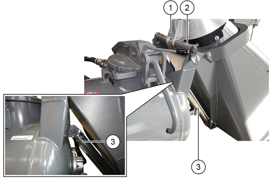
Şekil 78: Besleyici (B, BS) yağlama yerleri
