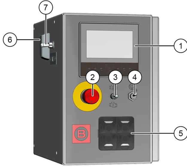
Şekil 15: Kumanda dolabı
