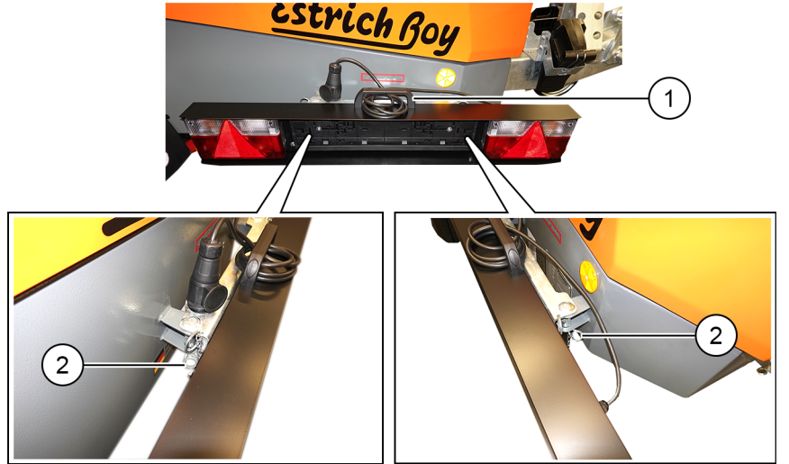
Şekil 32: Aydınlatma tertibatı
